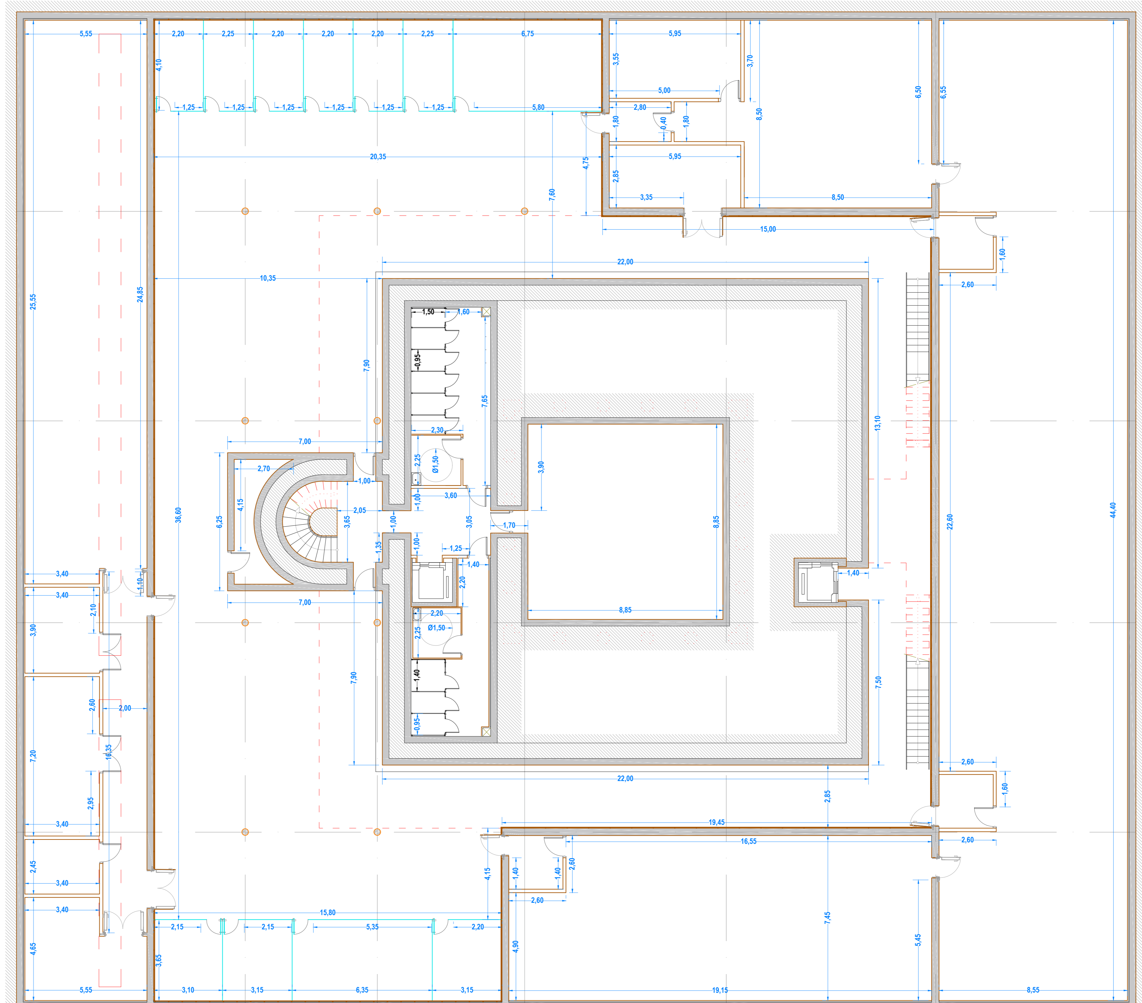
P. SÓTANO
